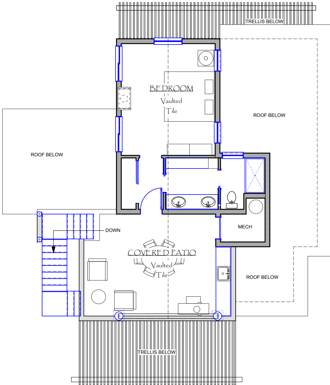
2 A1 UPPER FLOOR PLAN Scale: 1/8" = 1'-0"
