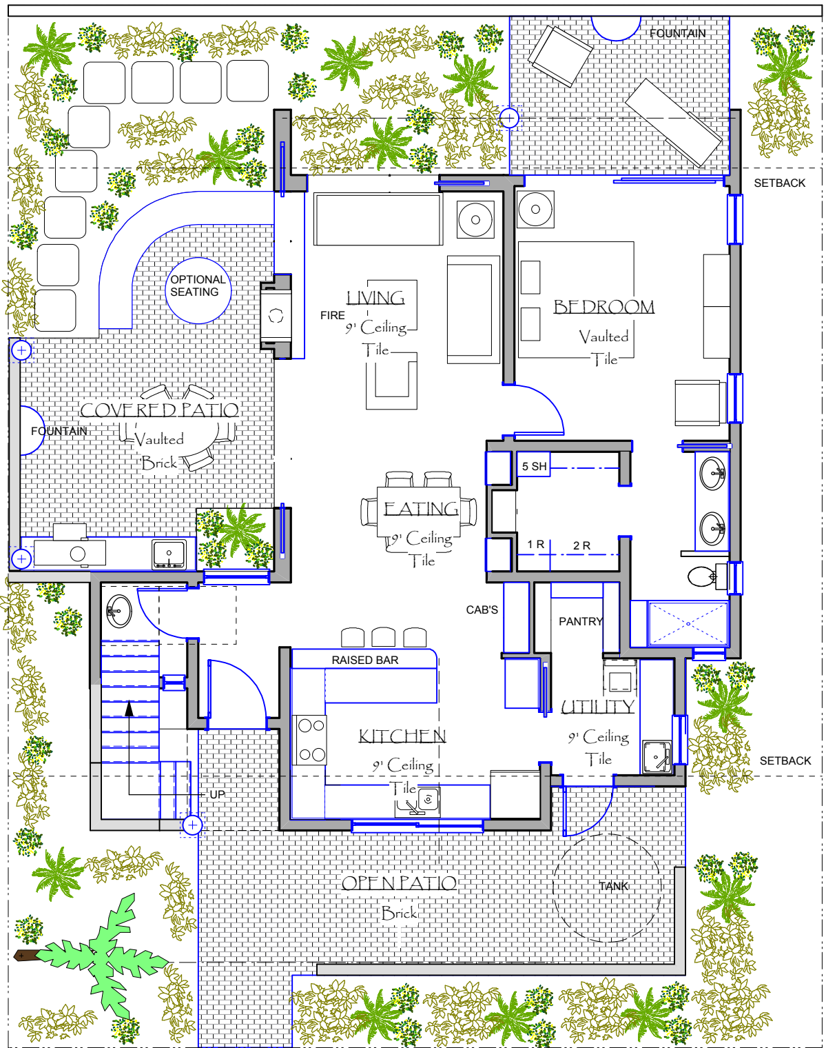
1 MAIN FLOOR PLAN A2 Scale: 1/8" = 1'-0"
